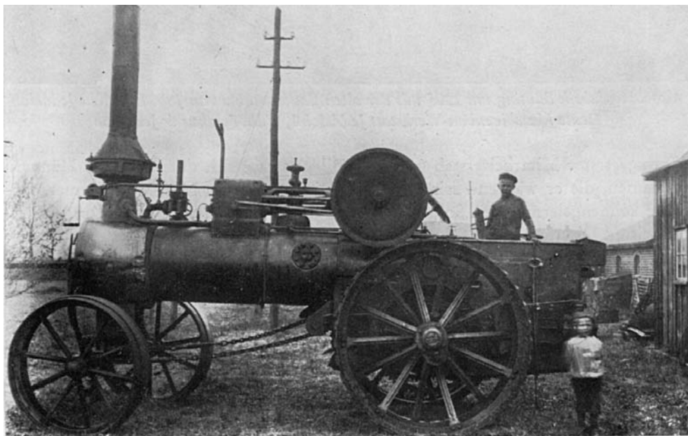
Edewechts erstes Dampflokomobil von Gerh. Bünting in Jeddelloh I – dahinter einer der ersten Gleichstrom-Lichtmasten des Bünting'schen Elektrizitätswerkes. Dieses Dampflokomobil diente anfänglich für das mit dem Betrieb ebenfalls verbundene Lohndreschunternehmen.
